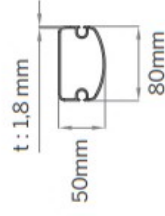
④ krajní vyztužovací profil
